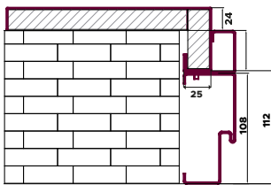
Opaska z ościeżnicą regulowaną IRON
