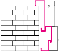
Opaska z ościeżnicą wewnętrzną IRON
