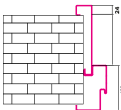
Opaska z ościeżnicą regulowaną IRON
