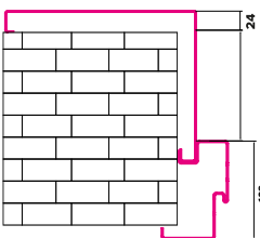
Portal z ościeżnicą regulowaną IRON
