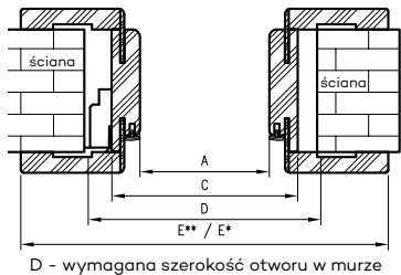
Przekrój poziomy OR/ORC
